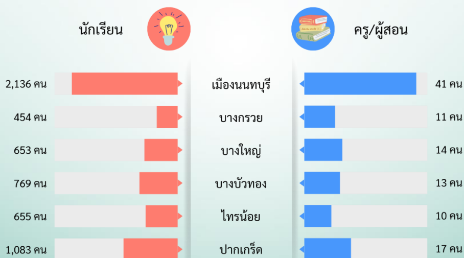
แผนภาพ 3 ข้อมูลนักเรียน ครู/ผู้สอน สังกัดสำนักงานส่งเสริมการเรียนรู้จังหวัดนนทบุรี
