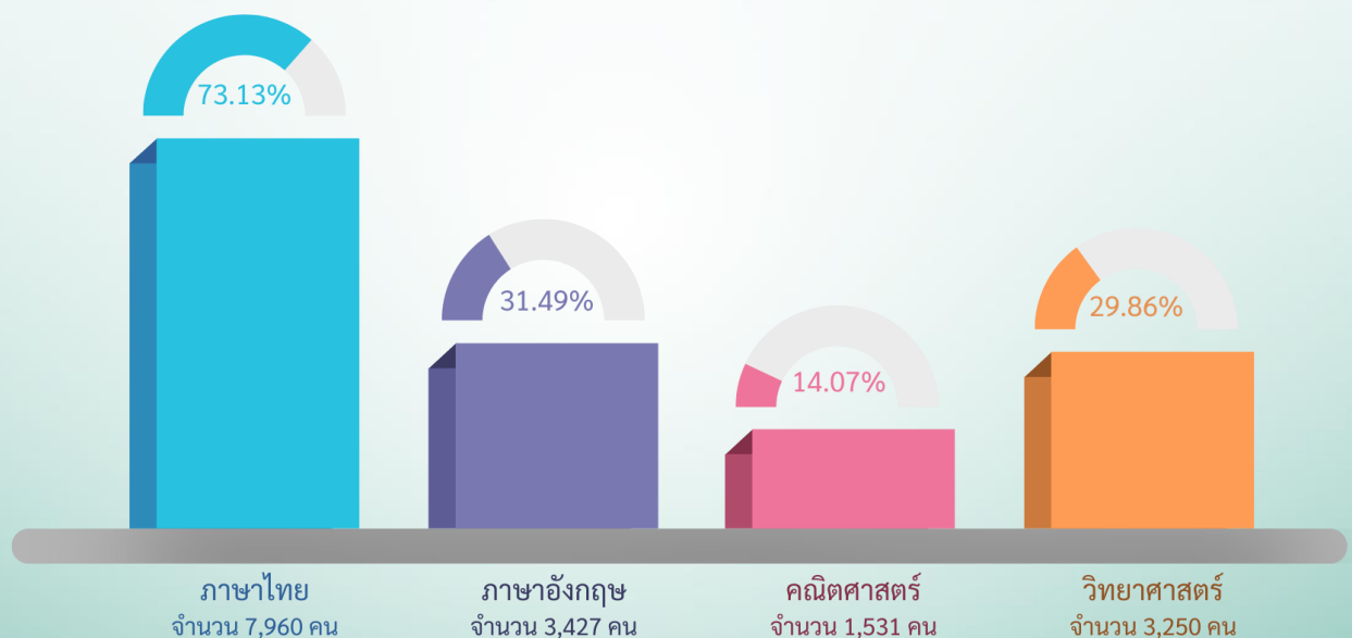
แผนภาพ 20 ร้อยละจำนวนนักเรียนระดับชั้นประถมศึกษาปีที่ 6 ที่มีผลคะแนน O-NET ผ่านเกณฑ์ ร้อยละ 50 ขึ้นไป
