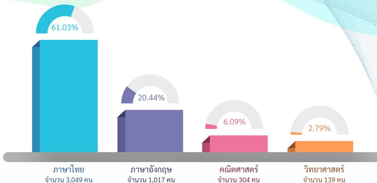
แผนภาพ 21 ร้อยละจำนวนนักเรียนระดับชั้นมัธยมศึกษาปีที่ 3 ที่มีผลคะแนน O-NET ผ่านเกณฑ์ ร้อยละ 50 ขึ้นไป
