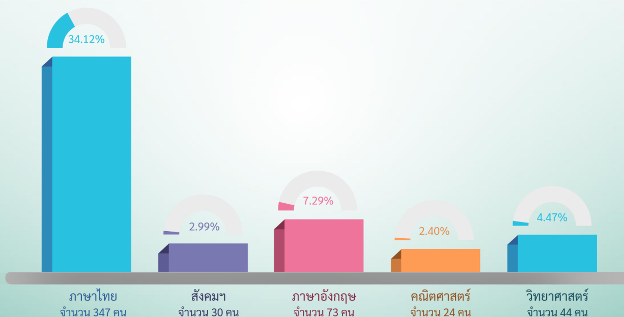
แผนภาพ 22 ร้อยละจำนวนนักเรียนระดับชั้นมัธยมศึกษาปีที่ 6 ที่มีผลคะแนน O-NET ผ่านเกณฑ์ ร้อยละ 50 ขึ้นไป
