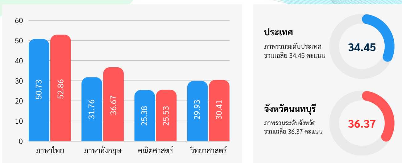
แผนภาพ 16 ผลการทดสอบ O-NET คะแนนเฉลี่ยชั้นมัธยมศึกษาปีที่ 3 ปีการศึกษา 2566
