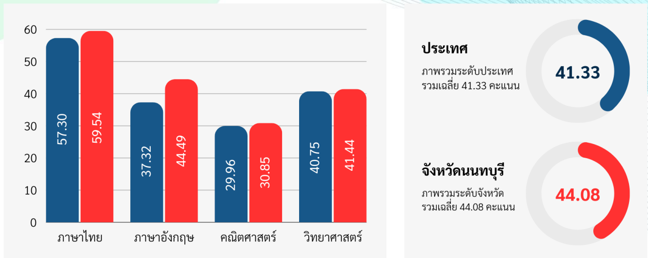
แผนภาพ 14 ผลการทดสอบ O-NET คะแนนเฉลี่ยชั้นประถมศึกษาปีที่ 6 ปีการศึกษา 2566
