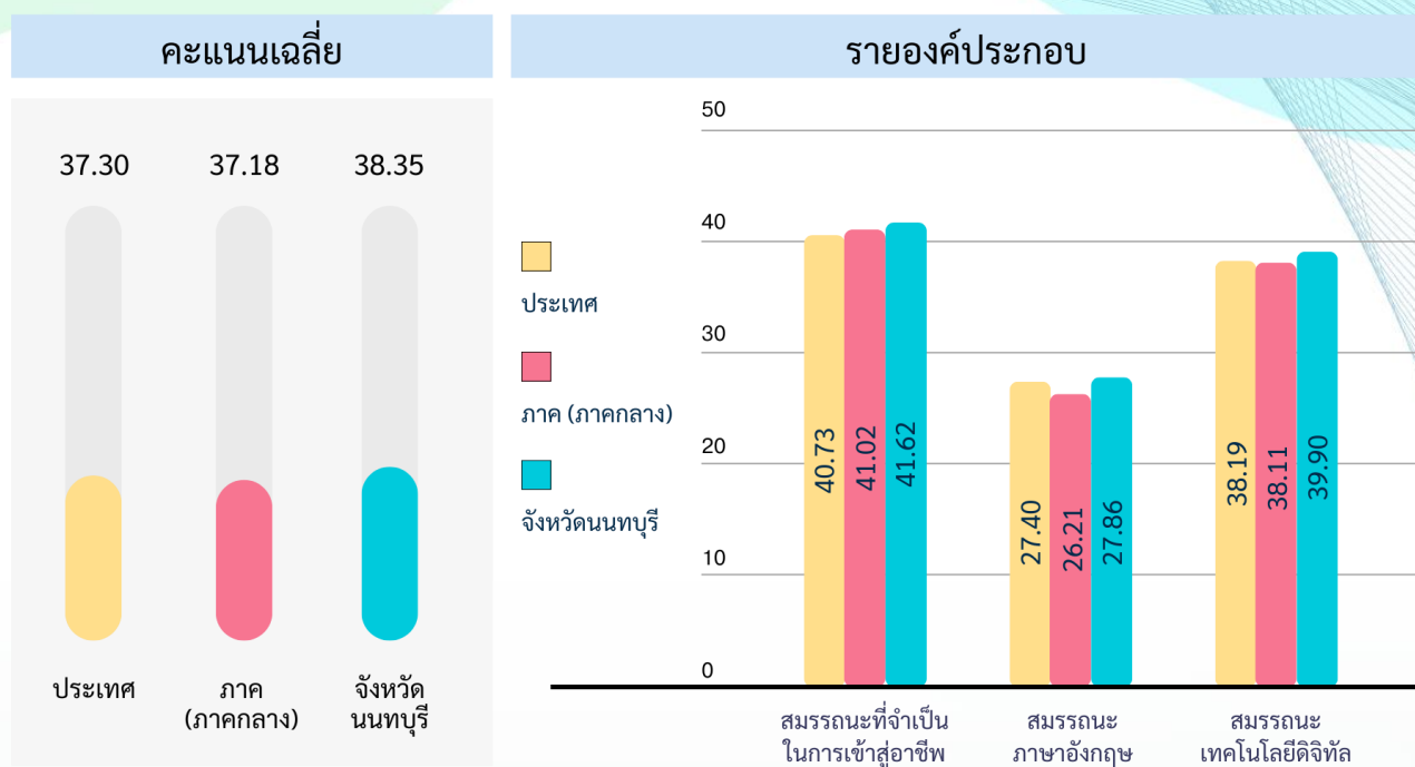
ดัชนีที่ 14 คะแนนเฉลี่ยผลการทดสอบทางการศึกษาระดับชาติด้านการศึกษานอกระบบโรงเรียน (N-NET)
