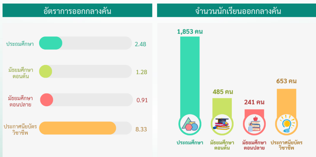
แผนภาพ 26 อัตราการออกกลางคันของนักเรียน จังหวัดนนทบุรี ปีการศึกษา 2566
