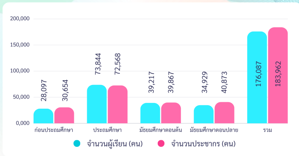
แผนภาพ 6 ร้อยละผู้เรียนเปรียบเทียบกับประชากรกลุ่มอายุ จังหวัดนนทบุรี
