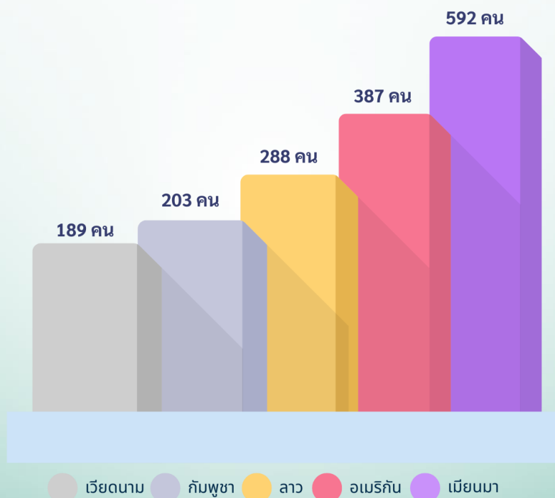
แผนภาพ 5 จำนวนผู้เรียนที่ไม่มีหลักฐานทางทะเบียนราษฎร (G-Code) จำแนกรายสัญชาติหรือชาติพันธุ์ ในพื้นที่จังหวัดนนทบุรี มากที่สุด 5 สัญชาติ/ชาติพันธุ์
